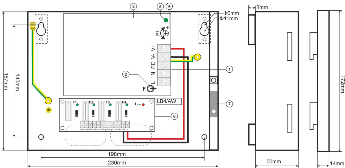
Rys.3. Widok zasilacza.
